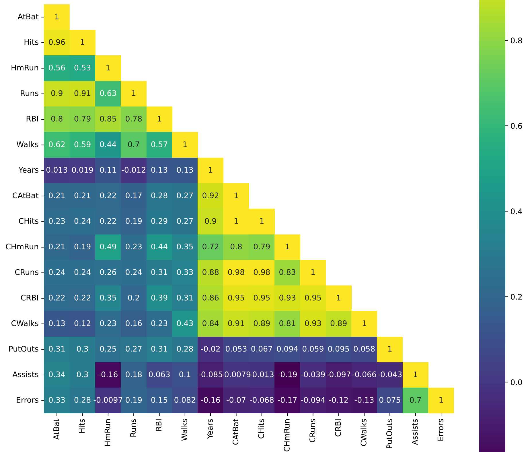
Correlacion de Pearson entre las Xs
